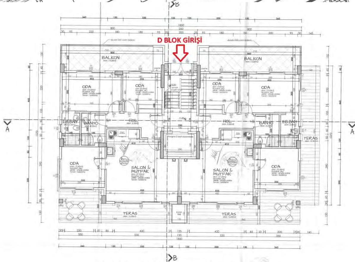
ZEMİN KAT PLANI Ö: 1/50
