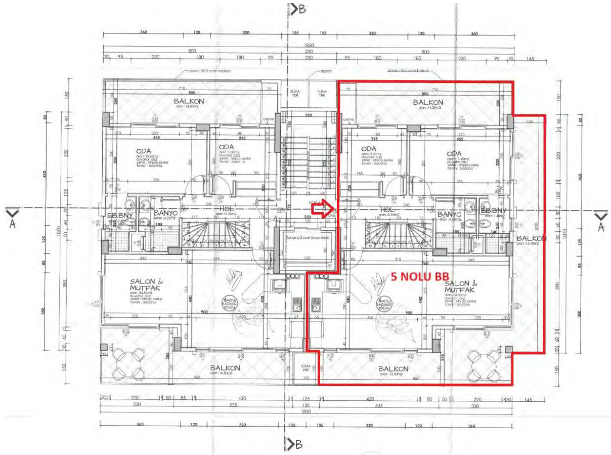
2. KAT PLANI Ö: 1/50
