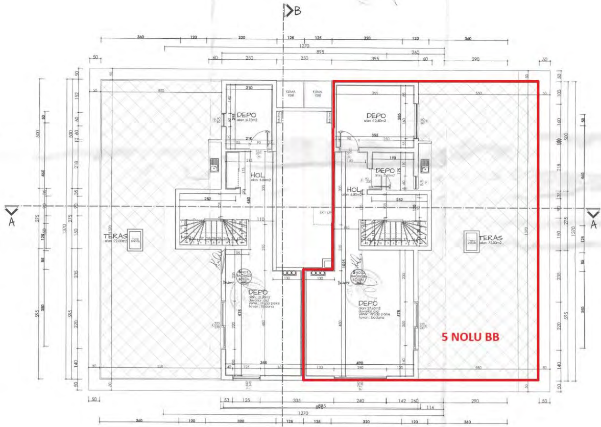
ÇATI KATI PLANI Ö: 1/50
